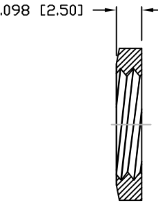
NUT
