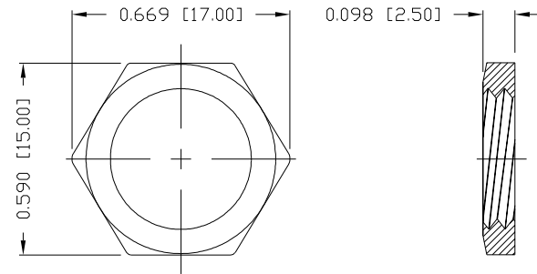
NUT
