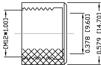
NUT
